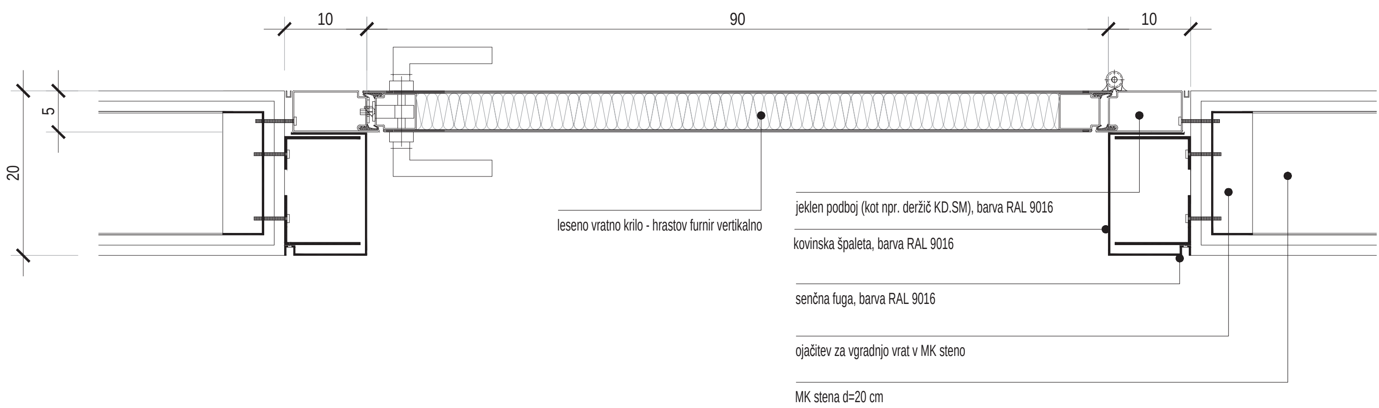
PRIKAZ VGRADNJE LESENIH VRAT S KOVINSKIM OKVIRJEM V MK STENO d=20cm
