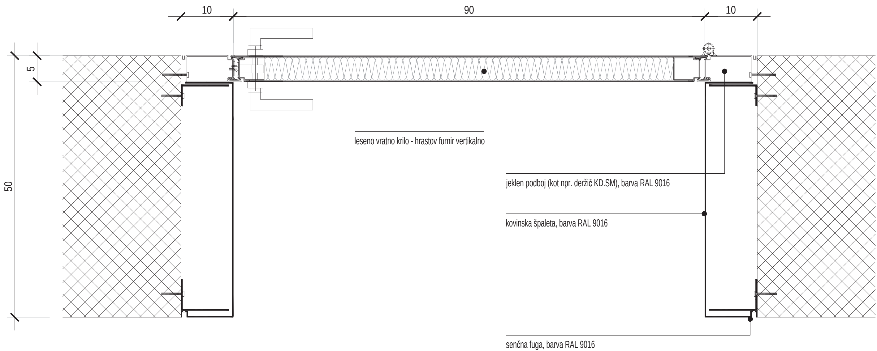
PRIKAZ VGRADNJE LESENIH VRAT S KOVINSKIM OKVIRJEM V AB steno d=25cm
